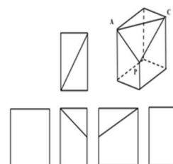
機械製図 (投影法)
